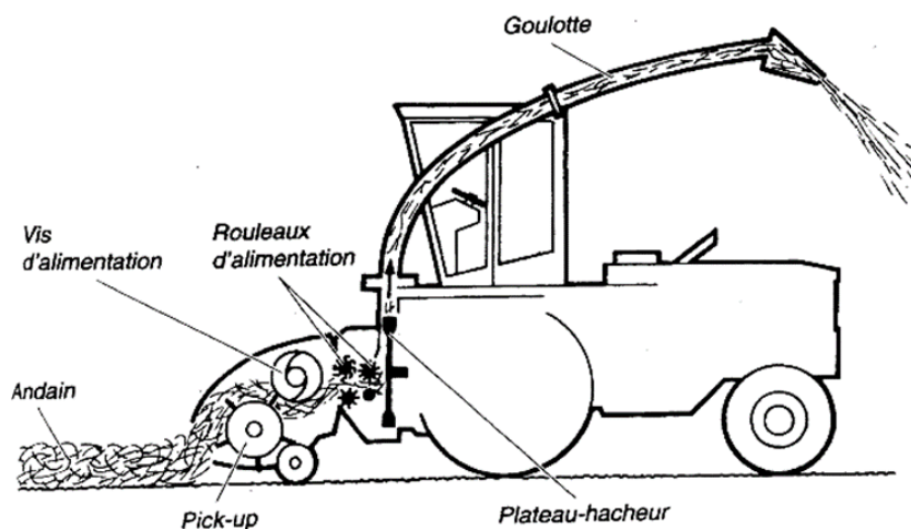
Figure 41 - Ensileuse automotrice (Anonyme dans Robberts H., 2002)
