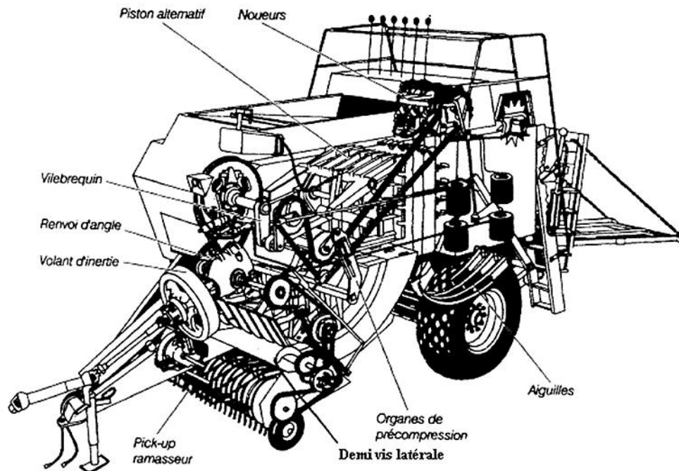
Figure 40 - . Presse à balles carrées (Anonyme dans Robberts H., 2002)
