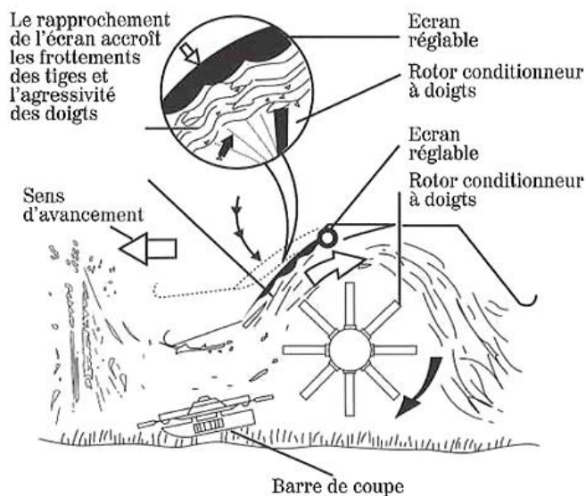
Figure 35 - Système de conditionnement à doigts (D'après Cédra, 1995 dans Vignau-Lousteau, 2008)
