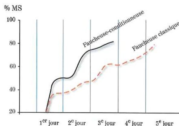
Figure 34 - Comparaison de la vitesse de séchage en fonction du type de faucheuse utilisée (Arvalis, 2003 dans Vignau-Lousteau, 2008)
