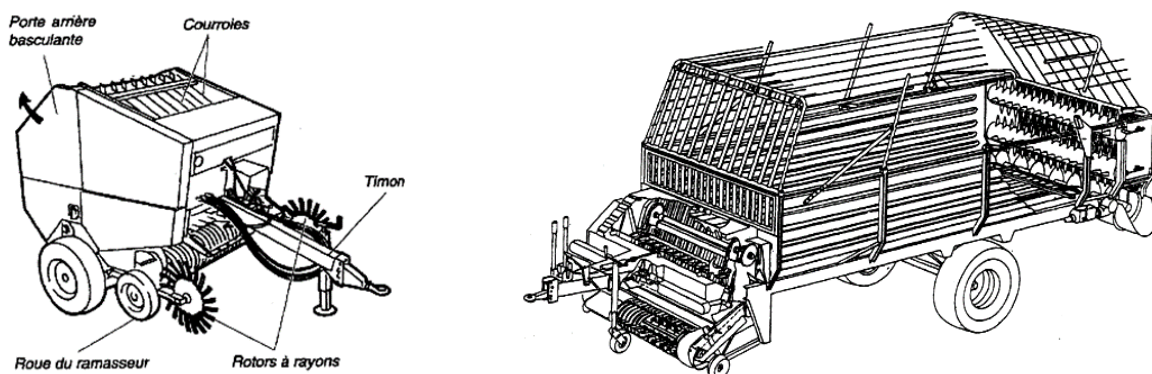
Figure 39 - Presse à balles rondes et remorque auto-chargeuse (Anonyme dans Robberts H., 2002)
