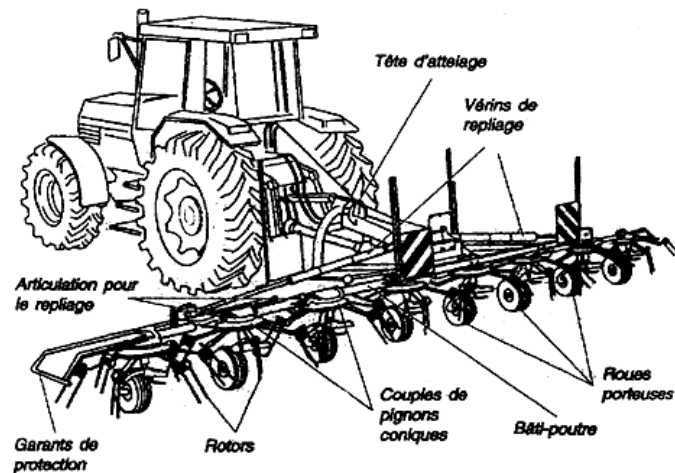
Figure 37 - Faneuse à toupies (Anonyme dans Robberts H., 2002)
