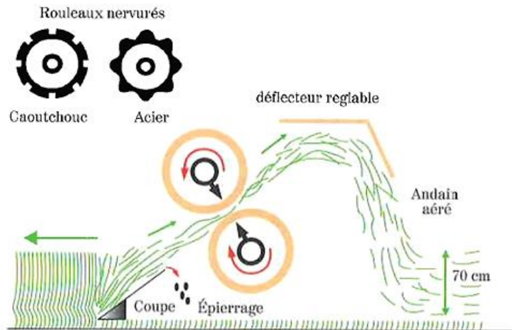
Figure 36 - Système de conditionnement à rouleaux (D'après Arvalis, 2003 dans Vignau-Lousteau, 2008)
