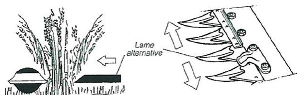
Figure 24 - Coupe par cisaillement (D'après Cédra, 1995 dans Vignau-Lousteau, 2008)
