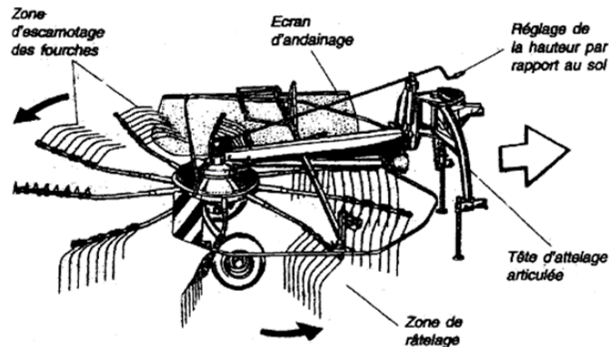
Figure 38 - Andaineur monorotor (Anonyme dans Robberts H., 2002)
