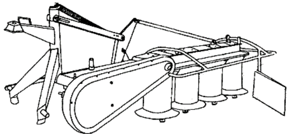
Figure 27 - Faucheuse à tambours (Detraux F. et Oestges O., 1979)
